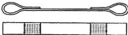
Рис. 1. Одиночный петлевой строп с мягкими плоскими петлями
