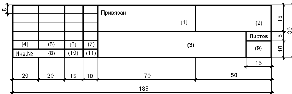
Штамп привязки (первый лист)
